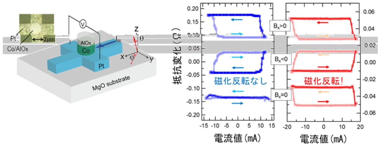
図 1. (a)単結晶 Co/Pt 磁化反転素子の模式図と(b)多結晶および単結晶 Co を用いた場合のスピン注入磁化反転結果。単結晶 Co/Pt 構造のみ外部磁場なし( B_x=0 )で磁化反転している。
