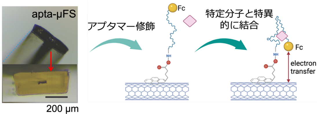
図 2. 多機能ファイバ技術とアプタマー技術の融合。カーボンナノチューブ (CNT) 複合材料を用いた電極ファイバの上にアプタマーを固定することにより、脳内の化学物質を特異的にセンシングすることが可能になった。
