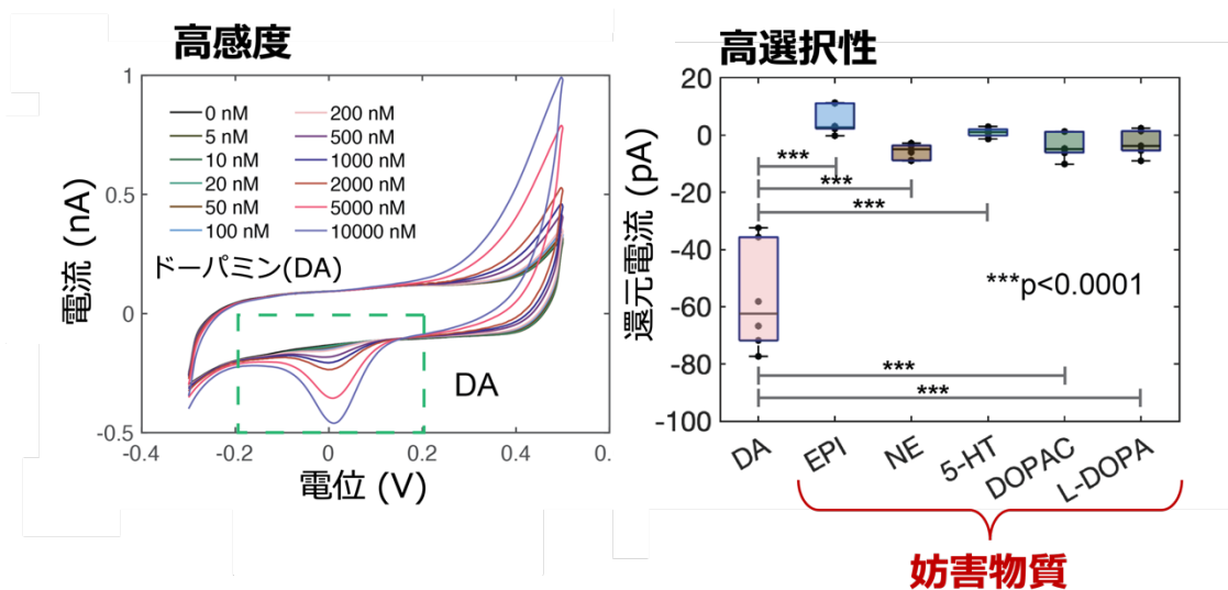
図 3. 今回開発したアプタマーファイバセンサによる、脳内の神経伝達物質であるドーパミン (DA) の測定結果。5nM までの低濃度のドーパミンの検出を実現した (左図) だけでなく、体内に共存するアスコルビン酸 (AA) や尿酸 (UA) などの主要妨害物質に対して高い特異性を示した。さらに、ドーパミンの前駆体であるレボドパ (L-DOPA)、その代謝物である 3,4-ジヒドロキシフェニル酢酸 (DOPAC)、モノアミン神経伝達物質のエピネフリン (EPI)、ノルエピネフリン (NE)、セロトニン (5-HT) といった類似構造を持つ化学物質を区別して検出できることを確認した (右図)。
