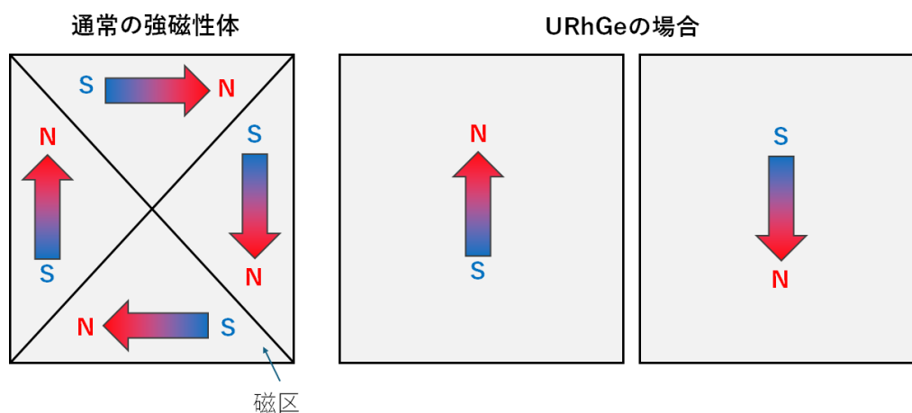
参考図表 2: 強磁性体 (Ferromagnetic) の作る磁区 (Magnetic domains)。通常 (Normal) の強磁性体では、左図のように磁気モーメントの揃う向きが異なる領域 (磁区) が物質内部で形成されます。磁区が形成されると、圧磁効果 (Magnetostriction effect) の観測が非常に困難になります。一方 URhGe は右図のように磁区 (Magnetic domains) を形成する傾向が非常に弱く、さらに磁気モーメントが \pm c 軸方向に向く傾向が強いというイジング性 (Ising-like) を持っているため圧磁効果 (Magnetostriction effect) が観測できたと推測しています。
