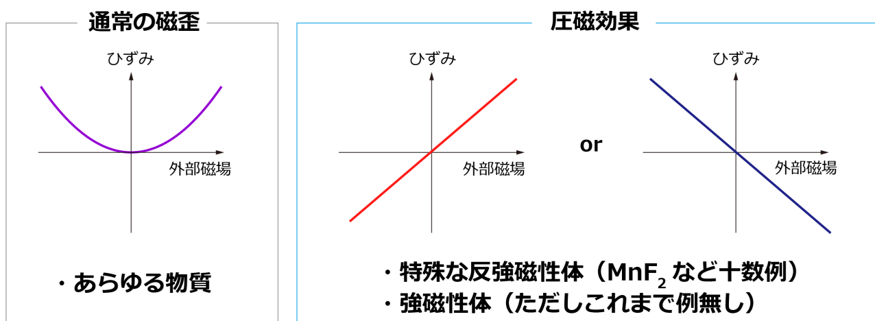
参考図表 1: 通常 (Normal) の磁歪と圧磁効果 (Magnetostriction effect) の比較。通常 (Normal) の磁歪では、左図のように外部磁場の 2 乗に比例するような磁場の正負に対して対称なひずみ-外部磁場曲線を示します。一方、圧磁効果は外部磁場の 1 乗に比例する効果で、右図のように直線的なひずみ-磁場曲線を示します。傾きの正負は磁気構造によって決まります。
