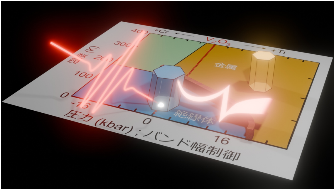
図 1.モット絶縁体 V_2O_3 の圧力-温度相図と本研究で行った「コヒーレントなひずみ波が誘起する結晶対称性変化」の模式図。 V_2O_3 は圧力や温度の変化によって構造が変化し、絶縁体や金属のように相が変化する。モット絶縁体（単斜晶、図中の黄緑色の立体）にフェムト秒レーザーパルス（図中赤色の振動波形）を照射することによって金属（菱面体、図中のオレンジ色の立体）への変化、すなわち絶縁体-金属転移が起きており、ひずみ波（圧力減少の波、図中白色の伝搬波形）のコヒーレント伝搬による高速な強弾性転移（単斜晶→菱面体）が起きていることがわかった。
