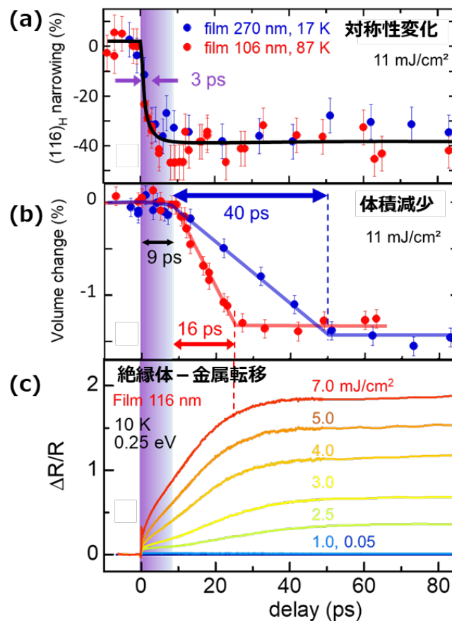
図 5. (a) 対称性変化 [(116) H 回折ピーク] の時間発展 赤：膜厚 106 nm、青：膜厚 270 nm。(b) 体積減少 [(110) H Bragg ピーク] の時間発展。(c) 絶縁体-金属転移 [過渡反射率変化 ( \Delta R/R )] の時間発展。
