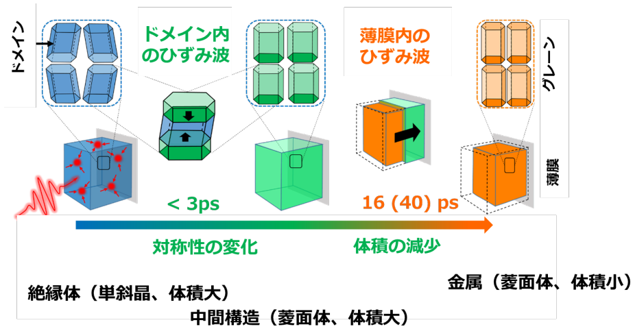
図 3. ひずみ波によるナノ結晶の光誘起構造変化のメカニズム。図中のモザイクタイル1ピースは、ナノ結晶（ドメイン: 平均粒径 20 nm）を表す。絶縁体（単斜晶、左側の水色の立体）にフェムトレーザーパルス（赤い振動波形）が照射されると、まず、単斜晶（水色）から菱面体（緑色）への対称性の変化が、ナノ結晶内の横波音波の伝搬として起こる。その後ナノ結晶の体積の減少が、ナノ結晶間の縦波音波（薄膜の厚さ方向）の伝搬として進行する（緑色→オレンジ色）。
