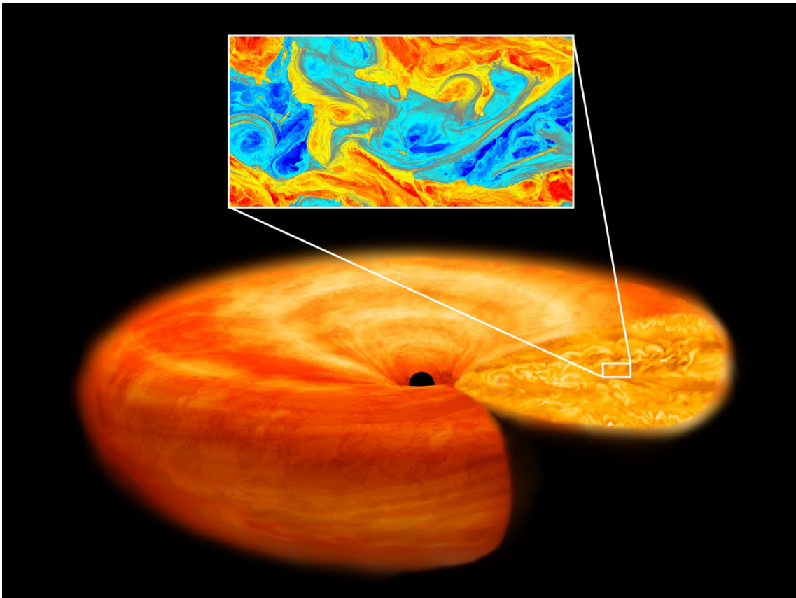
図 1. ブラックホール降着円盤のイメージ図と本研究で行った高解像度シミュレーションによって得られた磁場揺動分布。大きいスケールの渦が分裂していき、細かいランダムな渦構造が生まれる。(クレジット：川面洋平)
