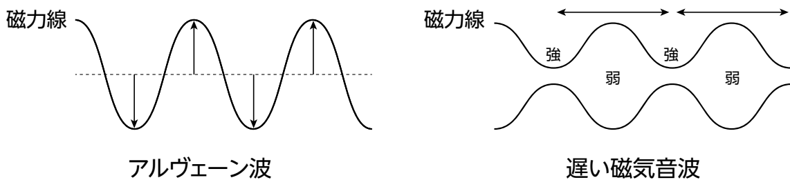
図 2. 降着円盤に存在する2種類の波 — アルヴェーン波（左）と遅い磁気音波（右） — の比較。アルヴェーン波は磁力線の振動を伴う横波で遅い磁気音波は磁場強度の強弱（すなわち磁力線間隔の粗密）が伝わる縦波。
