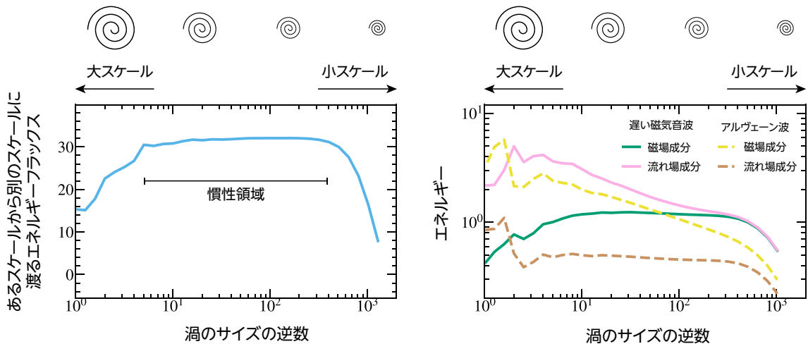
図 3. (左) あるスケールから別のスケールに渡るエネルギーフラックス。慣性領域では、この値は一定になる。この図では横軸の値が 4 から 400 程度まで一定値になっているので、慣性領域中の 100 倍大きさが違う渦を解像出来ていることになる。(右) あるスケールのゆらぎが持っているエネルギー。実線は遅い磁気音波、破線はアルヴェーン波。遅い磁気音波のエネルギーの方がアルヴェーン波のエネルギーより大きい（その差が約 2 倍）。また、横軸の値が 100 を超えたあたりから、遅い磁気音波注の磁場成分（緑）と流れ場成分（ピンク）が一致している。すなわち磁場エネルギーと運動エネルギーが当分配されている。
