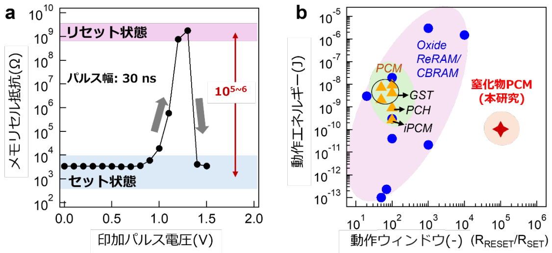
図 1. (a) 本研究で作製した記録素子の動作特性 (30ns の電圧パルスを用いて徐々に電圧を印加したところ、1.1V 付近にて低抵抗状態 (セット) から高抵抗状態 (リセット) へと変化し、1.4V 付近で再び低抵抗化するという、ナノ秒レベルの高速かつ不揮発な抵抗スイッチング挙動を示すことを発見した)。(b) 本研究の CrN メモリの動作エネルギーと動作ウィンドウのベンチマークプロット、および他の代表的な次世代不揮発性メモリとの比較 (注: ReRAM: 抵抗変化型メモリ; CBRAM: 導電性ブリッジメモリ; PCH: 相変化ヘテロ構造メモリ材料; iPCM (界面相変化材料))。
