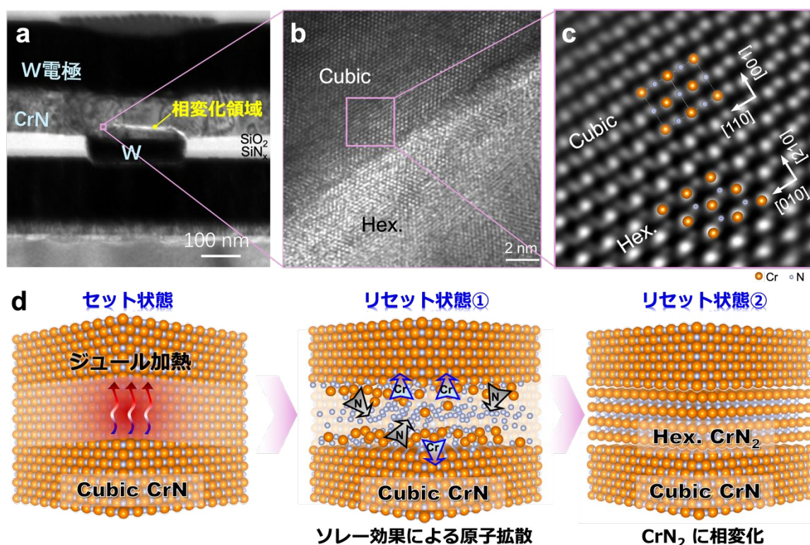
図 2. (a) 高抵抗状態にリセットされたデバイスの断面透過電子顕微鏡 (TEM) 画像。(b、c) 相変化領域境界で撮影された断面高分解 TEM 画像。(d) CrN の相変化における抵抗スイッチングメカニズムの概略図。
