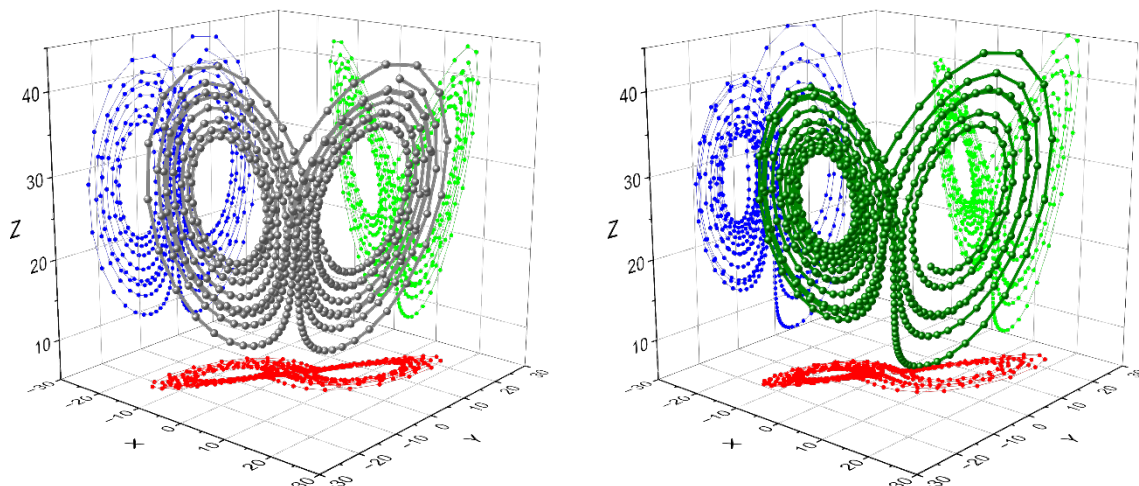
図 4. スピン波による物理リザーバ計算を用いたカオス時系列の予測。ローレンツモデルを用いて得られたカオス時系列の軌道を左図に示している。この時系列を用いて、ある時刻までのデータがある時に次の時間のデータを予測できるのかというタスクの学習を行った（右図）。カオス時系列は初期値鋭敏性があるために短時間の予測（短期予測）しかできないが、軌道自体は再現できることから、スピン波を用いた物理リザーバがモデルの構造を学習できていることを示唆している。
