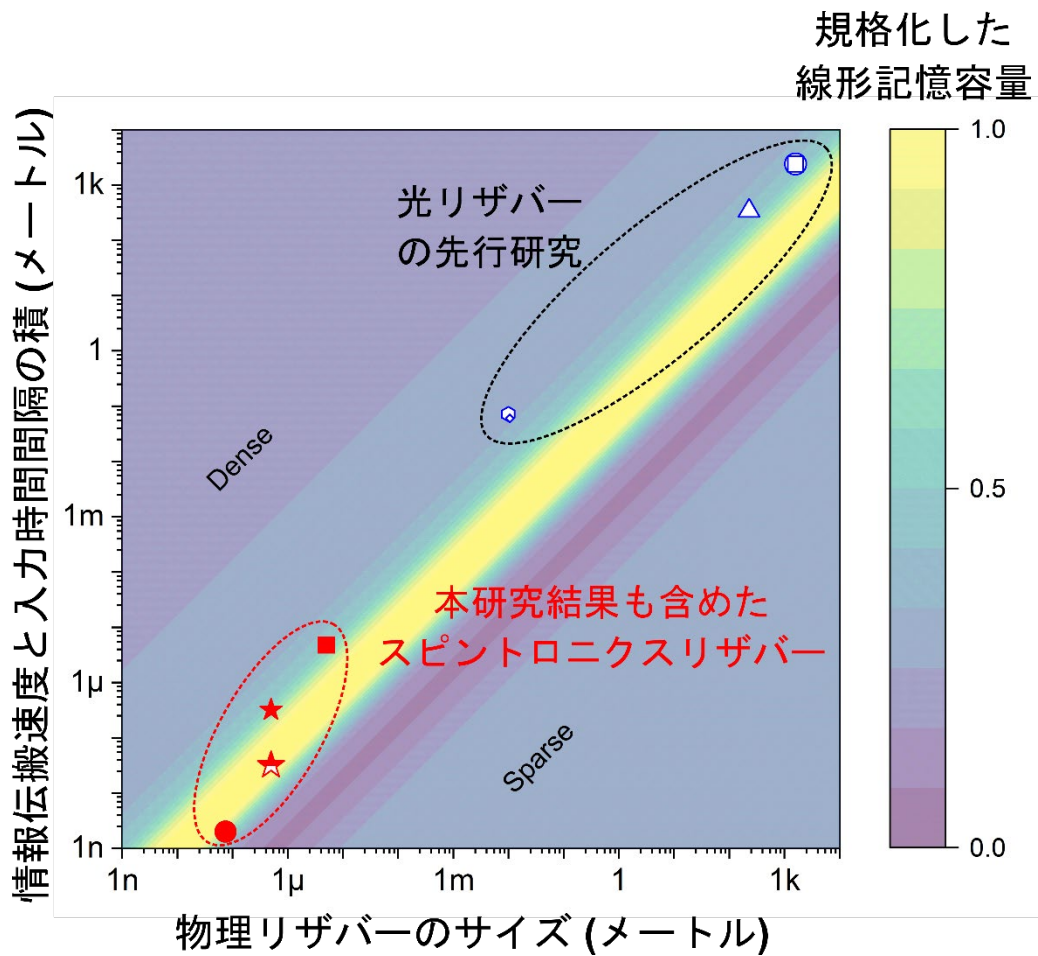
図 3. 最適な学習性能を実現するためには物理リザバーのサイズと情報伝播速度との間に条件が必要であることを数理的に解明した。本研究で、物理リザバーは、スピン波を用いるためにその伝播速度によってデバイスのサイズをサブマイクロ程度にすることができる。一方、光学素子を用いた系では、光速で情報が伝播されるため物理リザバーのサイズが大きくなってしまふ。
