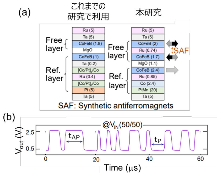
図 4. 従来研究を3桁上回る高速乱数生成動作が可能なスピントロニクス素子の膜構成(aの右側)と、今回作製したPビットが生成するランダムテレグラフノイズの測定結果(b)。
