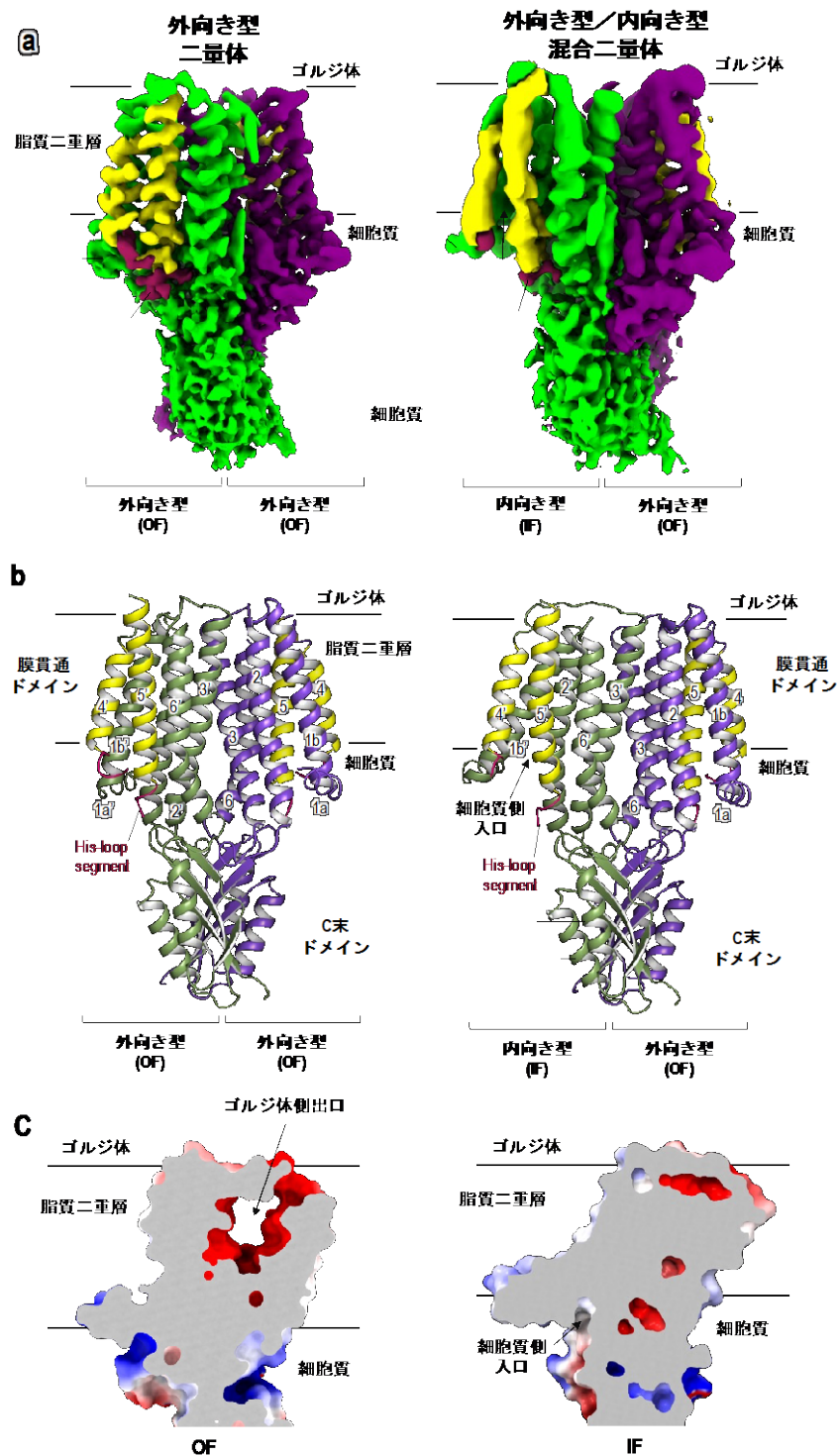
図 1. ZnT7 二量体のクライオ電子顕微鏡マップ (a)、分子構造モデル (b)、静電電荷マップの断面図 (c)。外向き型構造では、Golgi体側に亜鉛を放出する出口が形成される。一方、内向き型構造では、細胞質側から亜鉛を取り込むための入口が形成される。
