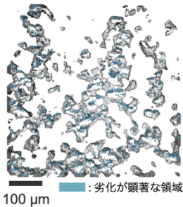
図 2.(a)3次元充電量マップの差分解析の模式図、(b)電極の劣化と、電極微細構造および反応履歴との相関分析の一例。
