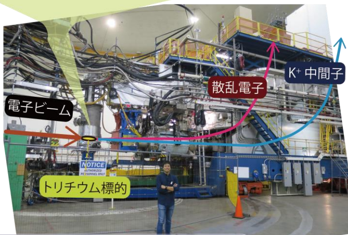
磁気分光器・HRS (左右二台) 米国・JLab
