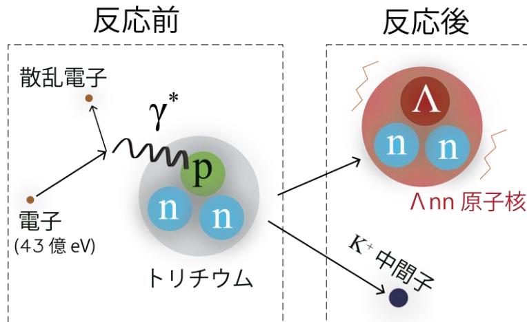
図 1 本実験で使用した反応の概念図。43 億電子ボルトに加速した電子を一秒間に 140 兆個 (140,000,000,000,000 個/秒) もの大強度でトリチウム標的に照射し、トリチウム中の陽子をラムダ ( \Lambda ) に変換しました。散乱された電子とこの原子核反応から生じた K^+ 中間子を検出器によってとらえて、 \Lambda nn 原子核の生成に起因する信号を調べました。
