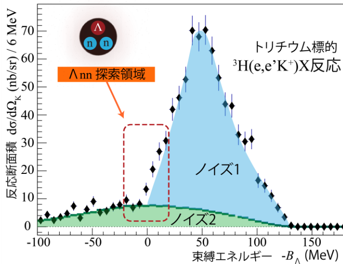
図 2 得られたエネルギースペクトラム。実際のデータは誤差棒付きの黒点で示しています。横軸のゼロ付近が \Lambda nn 原子核が存在すると期待される範囲で、本研究で信号探索を行いました。図中にノイズ 1、2 と示した領域はそれぞれシミュレーションや実データ解析で求められる信号以外 (背景事象) の大まかな領域です。これらの背景事象の分布を詳細に見積り、その背景事象の寄与を除いた後の「あまり」を \Lambda nn 原子核の信号の可能性のある事象として解析しました。
