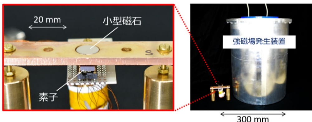
図2 (左)小型磁石を用いる新型量子抵抗標準素子と、(右)従来必要だった強磁場発生装置との比較
