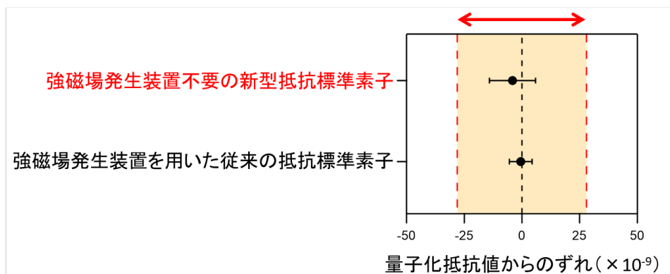
図3 新型抵抗標準素子、従来の抵抗標準素子それぞれで測定された抵抗値の量子化抵抗値からのずれ(相対値)。図中の矢印は産総研の抵抗校正における校正測定能力を実現可能な相対標準不確かさの大きさ( \pm 28 \times 10^{-9} )。
