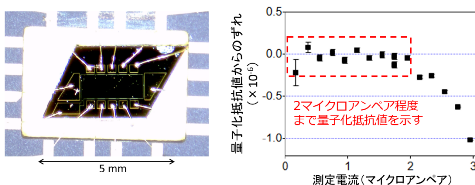
図 1 (左)トポジカル絶縁体を用いて作製した量子抵抗標準素子。(右)抵抗値の量子化抵抗値からのずれ(相対値)の測定電流依存性。
