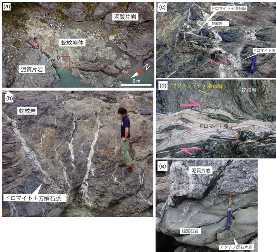
図1 露頭における樋口蛇紋岩体と炭酸塩脈(き裂を炭酸塩鉱物で充填されたもの)の産状。(a) 蛇紋岩体のドローン写真。(b-d) 蛇紋岩を切って発達する炭酸塩脈のネットワーク。(b) 脈の太い部分は主にドロマイト( \text{CaMg}(\text{CO}_3)_2 )や方解石( \text{CaCO}_3 )からできており、(c) ドロマイト+滑石脈で切られた蛇紋岩部分はマグネサイト( \text{MgCO}_3 ) + 滑石の細かい脈が含まれている。(d) 炭酸塩脈の構造は脈形成後に剪断変形を受けていることを示している。(e) 蛇紋岩体の境界部分では、堆積物起源の変成岩(泥質片岩)が緑泥石岩に変化しており、蛇紋岩体からマグネシウムが放出されたことを示している。
