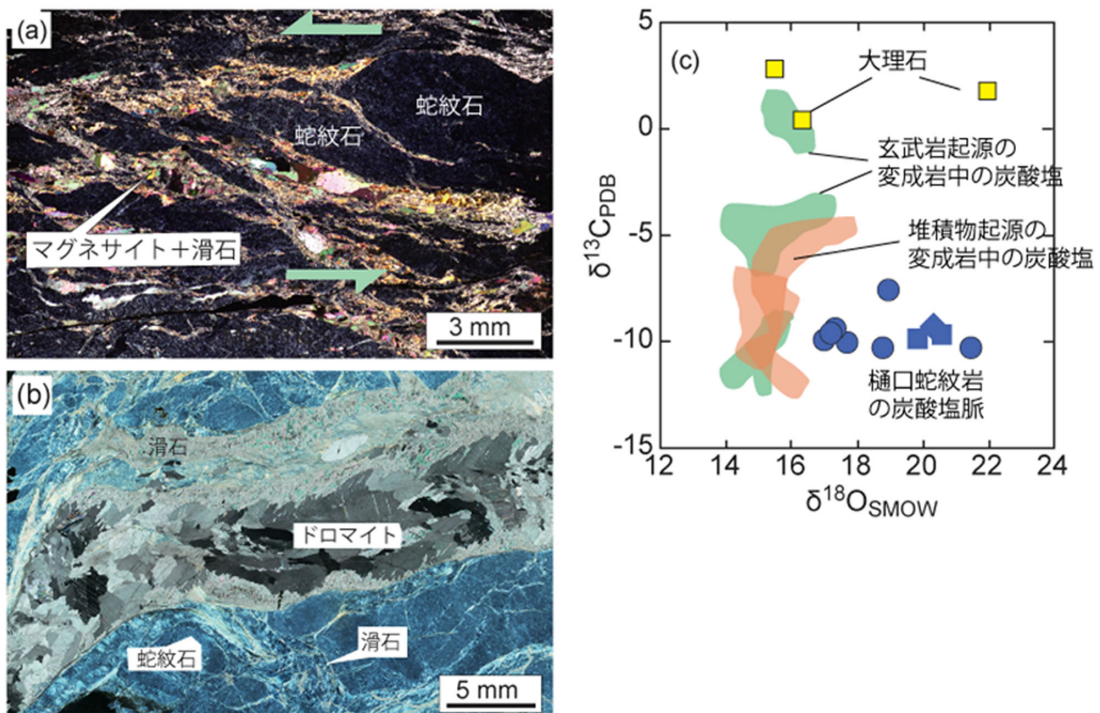
図2 樋口蛇紋岩体の炭酸塩脈の特徴。(a) 蛇紋石(アンチゴライト)のブロックを切るマグネサイト+滑石脈。蛇紋石ブロックの非対称の組織から剪断変形を受けていることがわかる。(b) ドロマイト+滑石脈。蛇紋石と二酸化炭素が反応する炭酸塩化反応では、シリカが放出されるために、シリカに富む層状ケイ酸塩鉱物である滑石ができる。滑石は変形しやすいやわらかい鉱物であり、プレート境界の性質を大きく変化させる。(c) 樋口蛇紋岩体の炭酸塩鉱物の炭素と酸素の安定同位体組成。三波川帯の中に出てくる大理石(海洋底で形成した炭酸塩が沈み込んだもの)とは大きく異なっている。蛇紋岩中の炭酸塩脈の炭素同位体は、堆積物起源の変成岩に含まれる炭酸塩とよく似ているが、酸素同位体はより高くなっており、堆積物中の炭素を起源とする二酸化炭素と蛇紋岩から脱水した水が混合したことを示唆している。
