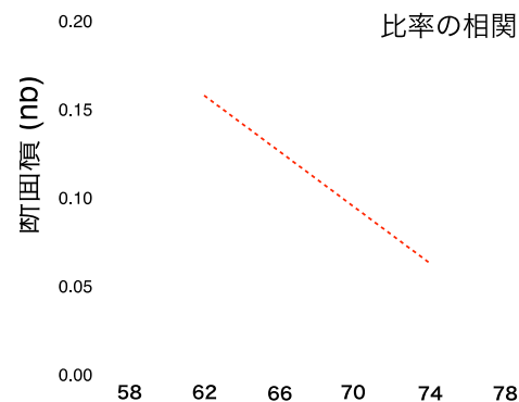
図3 原子核内のアルファ粒子生成を示す実験結果(左)と同位体依存性の実験結果と理論予想
