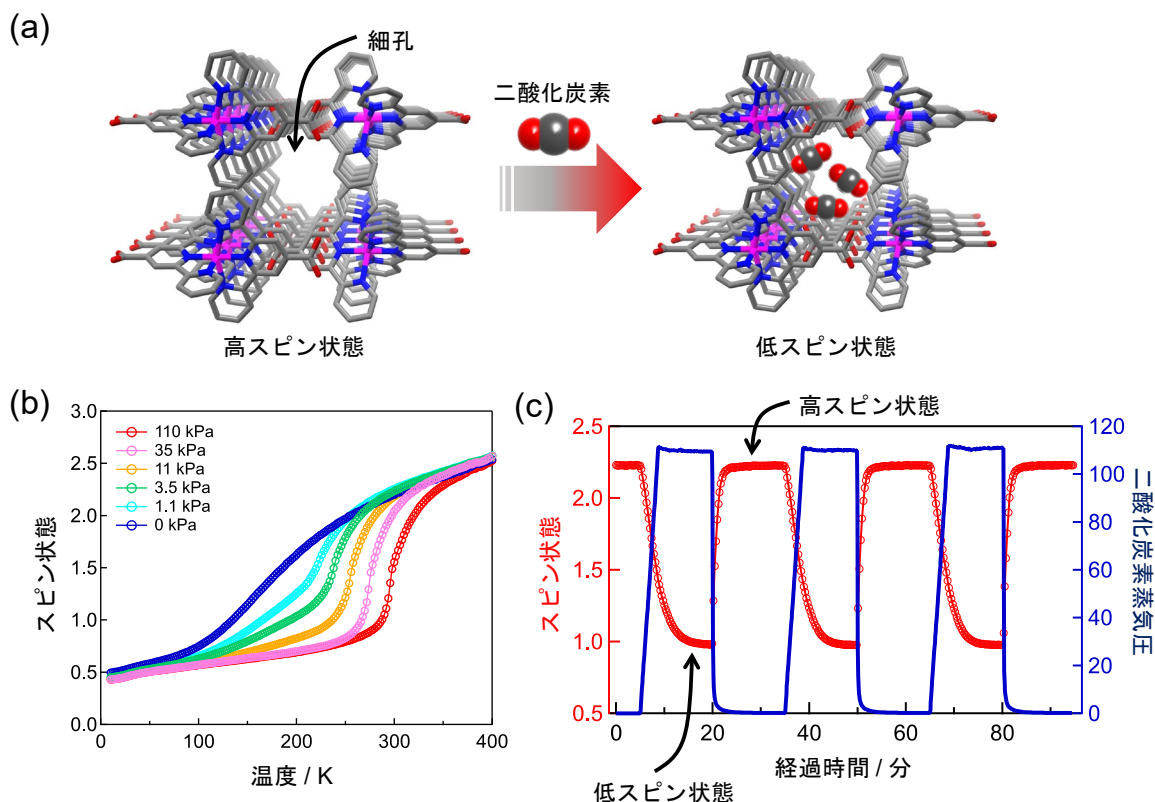
図 2. (a)脱水後のコバルト(II)錯体の細孔および二酸化炭素吸着の模式図。(b)二酸化炭素分圧によるスピントクロスオーバー特性の変化。(c)二酸化炭素吸脱着に伴う可逆的なスピン状態変換。
